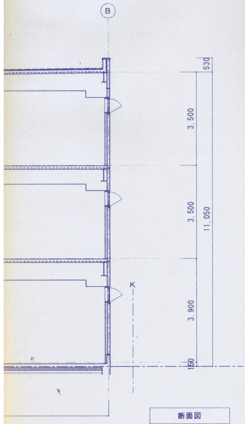
断面図
